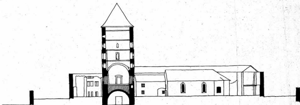
SECȚIE C-D
