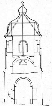
SECȚIA E.-VEST
