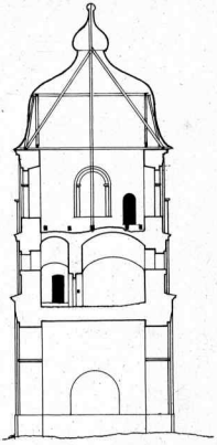
SECȚIA S.-NORD
