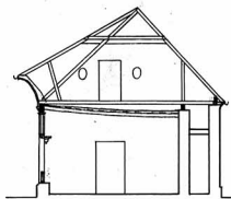
secție A-B
