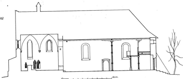
BISERICA LUTERANĂ DIN VALEA LUNGĂ - J. TÂRNAVA MICĂ - RELEVU II-1929 - ARHIT. J. C. 1929
