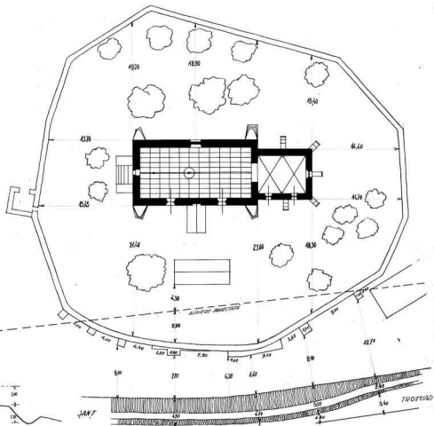
Biserica Luterană din Valea Lungă J. Târnava Mică JCARA 5 nr. - 41. RELEVU IX - 1949 ARHITECT J. J. J.
