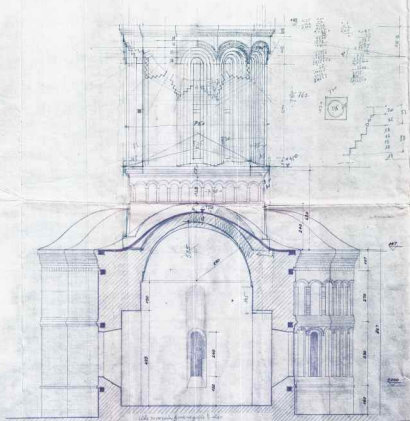
SECȚIUNE TRANSVERSALĂ
