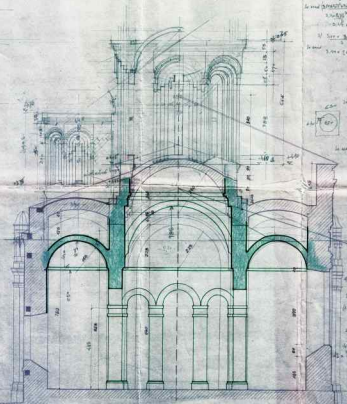
SECȚIUNE TRANSVERSALĂ PRIN FRONȚĂ - PROMIDERE ȘI BILEVU
