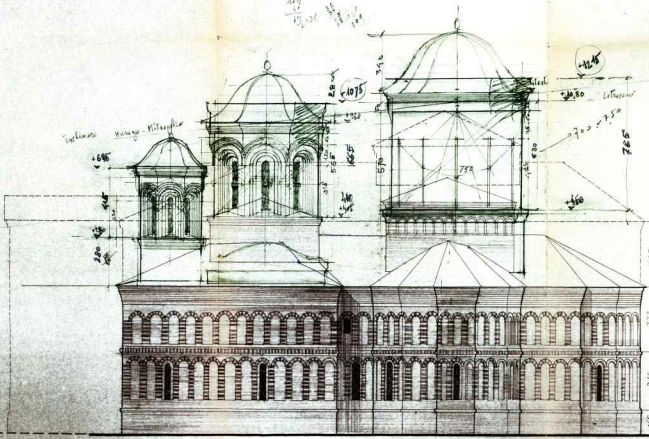
FATADA SUD VARIANTA III 1:100
