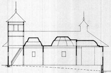
SECȚIUNE
