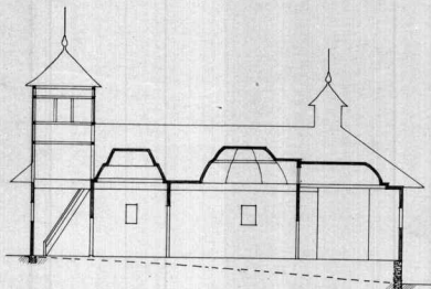
SECȚIUNE
