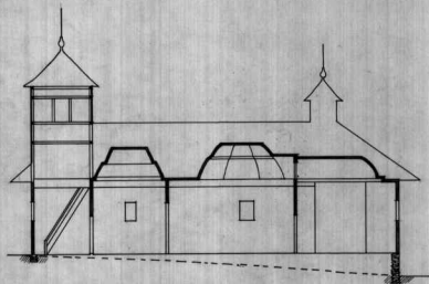
SECȚIUNE
